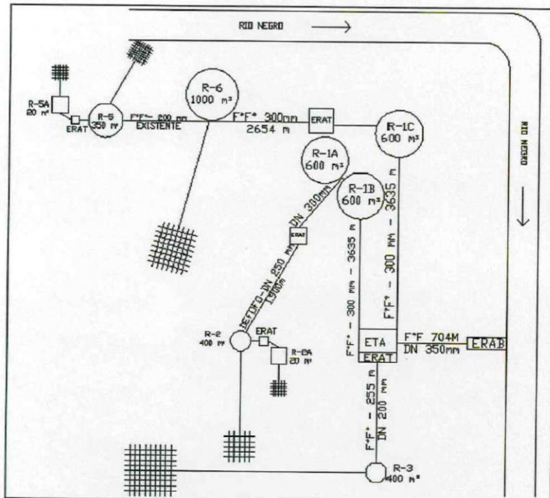
Figura 29 – Croqui do SAA de Mafra.
