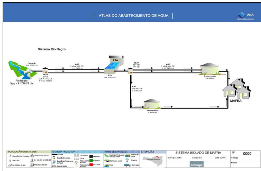
Figura 2 - Fluxograma do SAA de Mafra em Junho/2009
