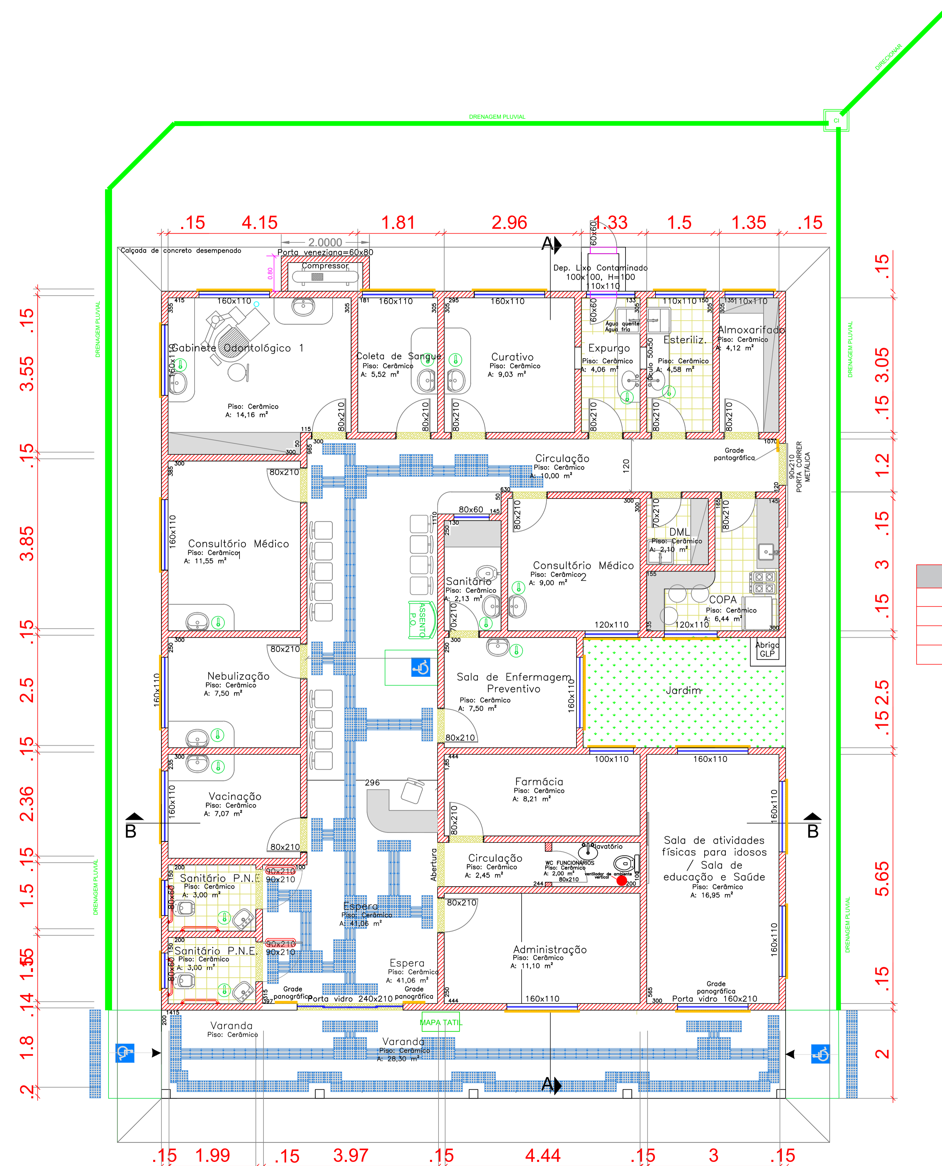
PLANTA BAIXA - ACESSIBILIDADE ÁREA: 247,47m 2 ESC 1/50
