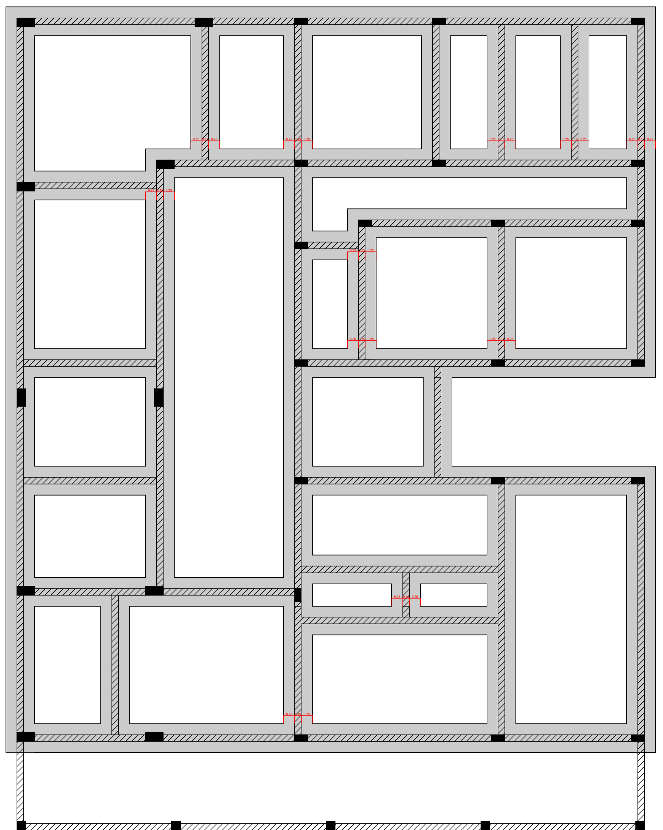
ÁREA DE INTERVENÇÃO - SAPATAS CORRIDAS ESC 1/50
